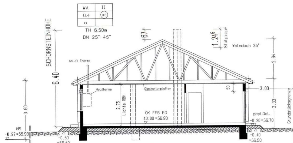
Grundriss EG und Schnitt gemäß Baugenehmigung
